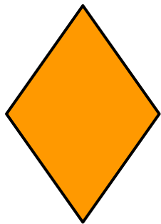
Rhombus
